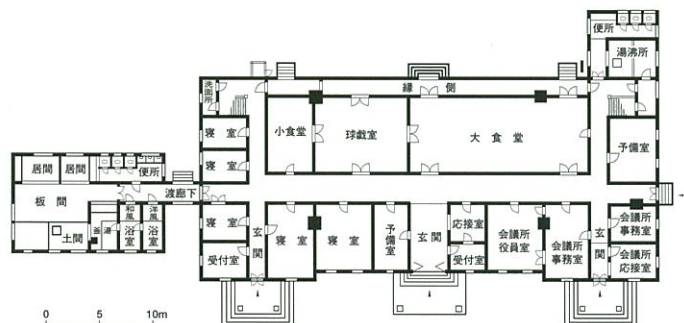
旧函館区公会堂一階平面図
